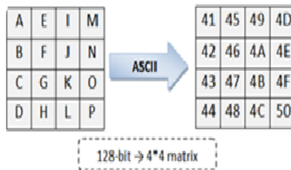
Fig. 1 ASCII Conversion
